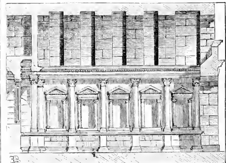
Fig. 493. Nymphæum at Nismes (restored).
